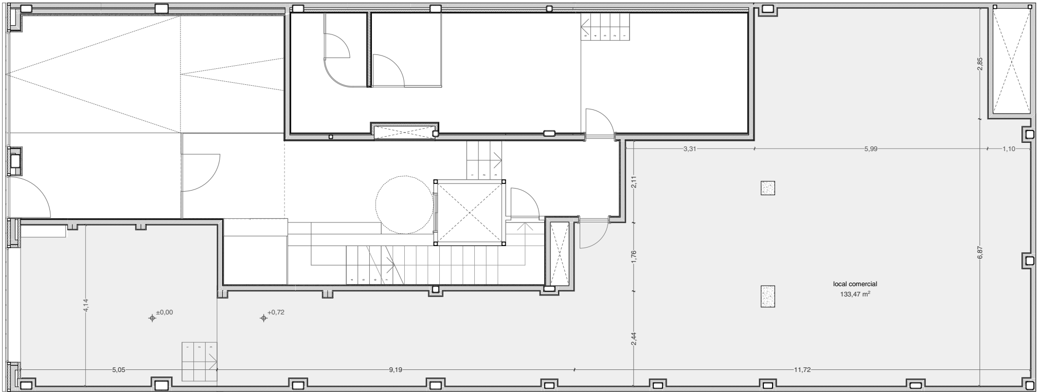
PLANTA BAJA_local comercial e: 1/100
